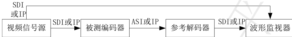
图10 视频技术指标测量框图
